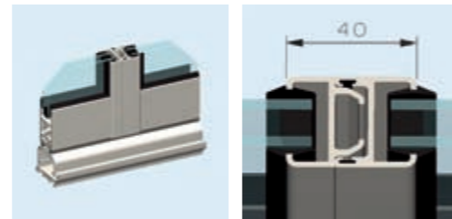
Filigrane Profilsicht 40mm | Filigree profile view 40mm | Vista filigrana del perfil de 40 mm
