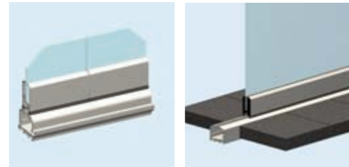
aufgesetzte Bodenschiene mit Entwässerungsrinne | bottom floor track with drainage channel | Guía inferior con un canal de drenaje
